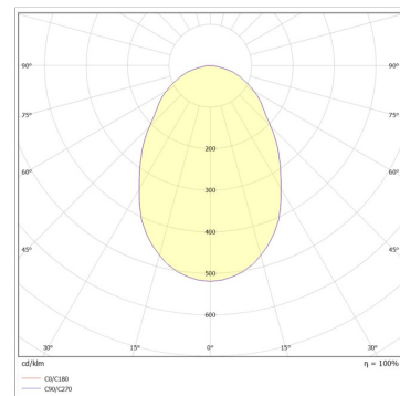
RDL AL G2 RGBW Polar Curve
